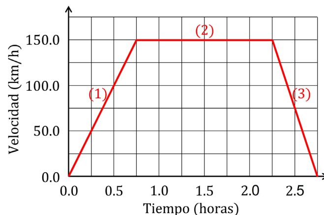
Figura 5: Descripción de la velocidad seguida por el cuerpo.
